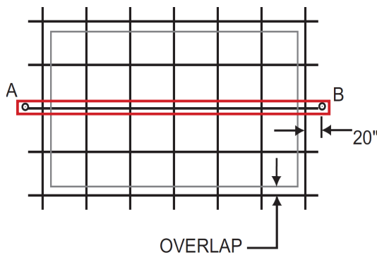
Install Center Strap A-B
